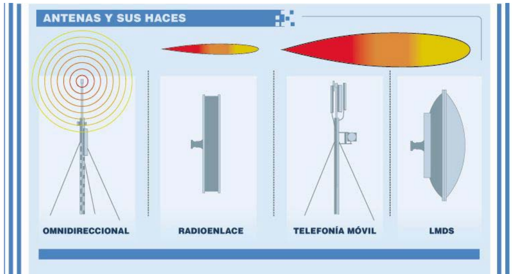
Figura nº 13. Diferentes tipos de antenas y sus haces de emisión. Fuente: Informe sobre Emisiones Electromagnéticas de los sistemas de Telefonía móvil y acceso fijo inalámbrico. Colegio Oficial Ingenieros Telecomunicación. 2001.
